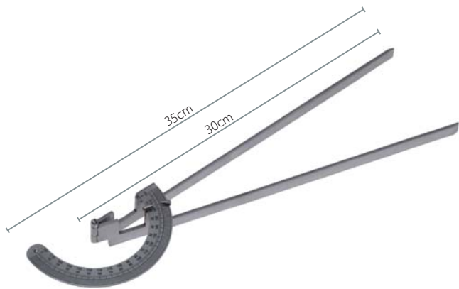
角度計 東大 Measuring Meltken Japan 商品コード Z813-153A サイズ 35cm 価格 ¥9,000
