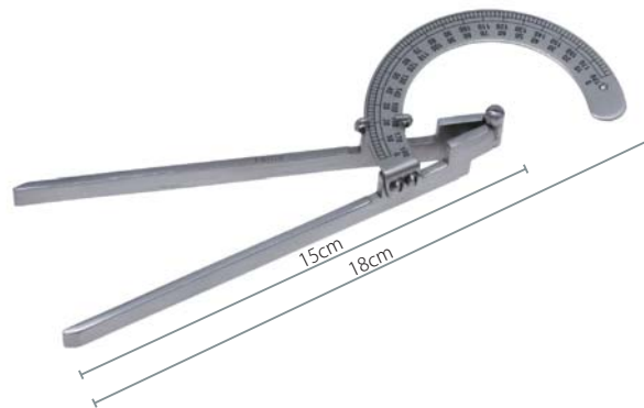
角度計 メルトゲン Measuring Meltken 商品コード Z813-153B サイズ 18cm 価格 ¥9,500
